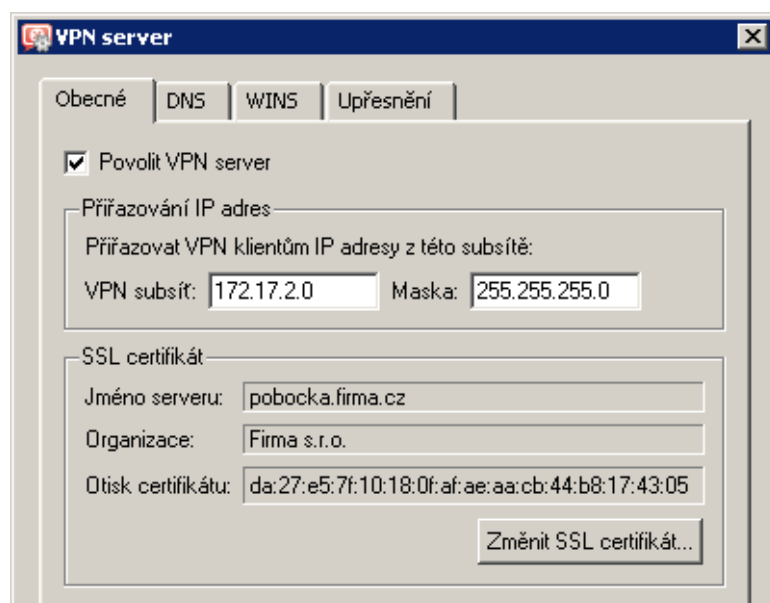
Obrázek 23.29 Pobočka — konfigurace VPN serveru
