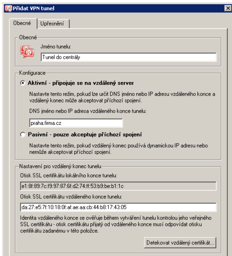
Obrázek 23.30 Pobočka — definice VPN tunelu do centrály
