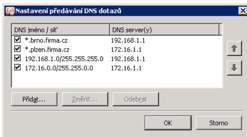
Obrázek 23.37 Centrála — nastavení předávání DNS dotazů
