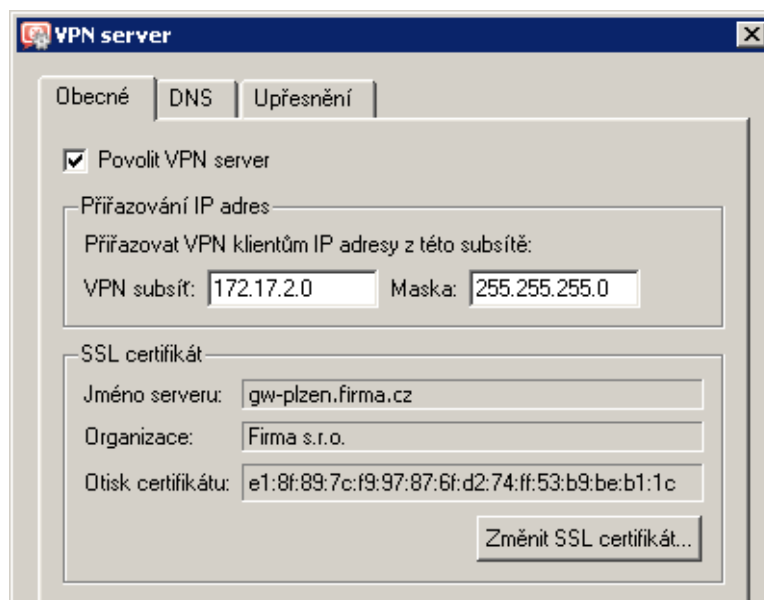
Obrázek 23.50 Pobočka Plzeň — konfigurace VPN serveru
