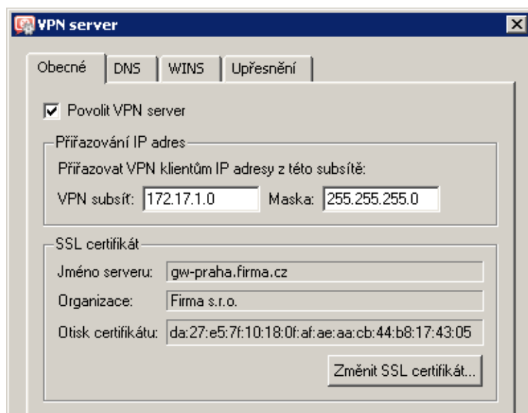
Obrázek 23.20 Centrála — konfigurace VPN serveru
