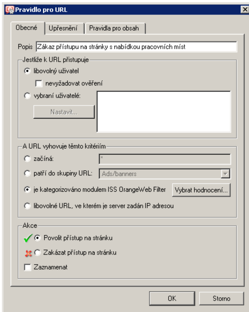
Obrázek 12.8 Pravidlo pro filtrování WWW stránek dle kategorií systému ISS OrangeWeb Filter
