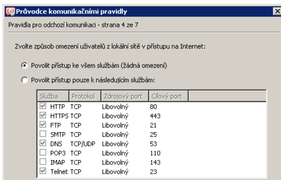
Obrázek 23.23 Pobočka — přístup z lokální sítě do Internetu bez omezení
