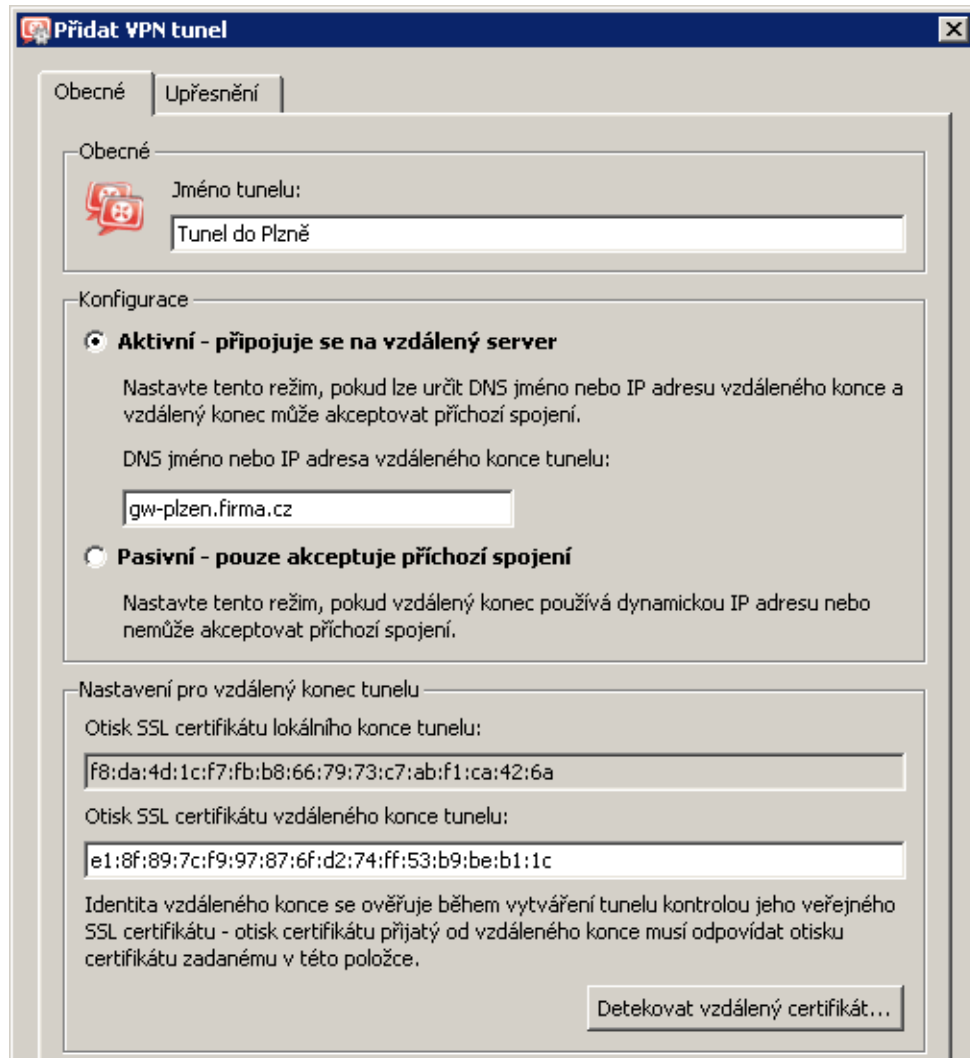
Obrázek 23.63 Pobočka Brno — definice VPN tunelu do pobočky Plzeň
