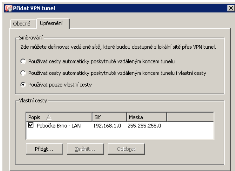
Obrázek 23.54 Pobočka Plzeň — nastavení směrování pro tunel do pobočky Brno
