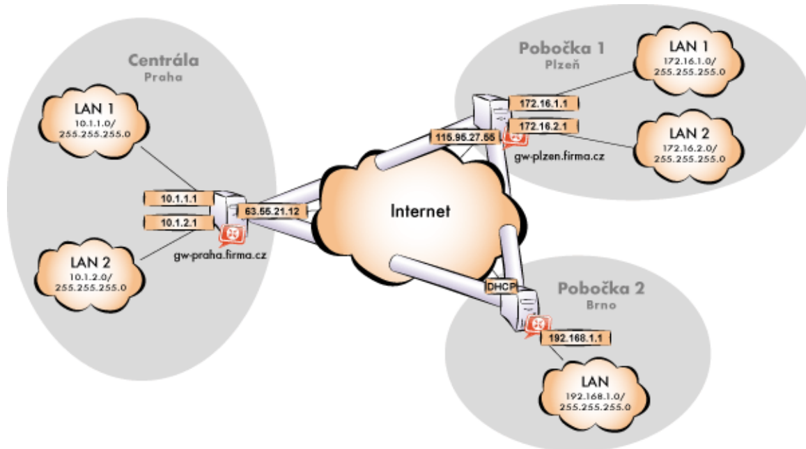
Obrázek 23.32 Příklad konfigurace VPN — firma se dvěma pobočkami
