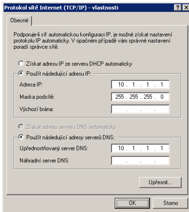
Obrázek 23.19 Centrála — konfigurace TCP/IP na rozhraní firewallu připojeném do lokální sítě
