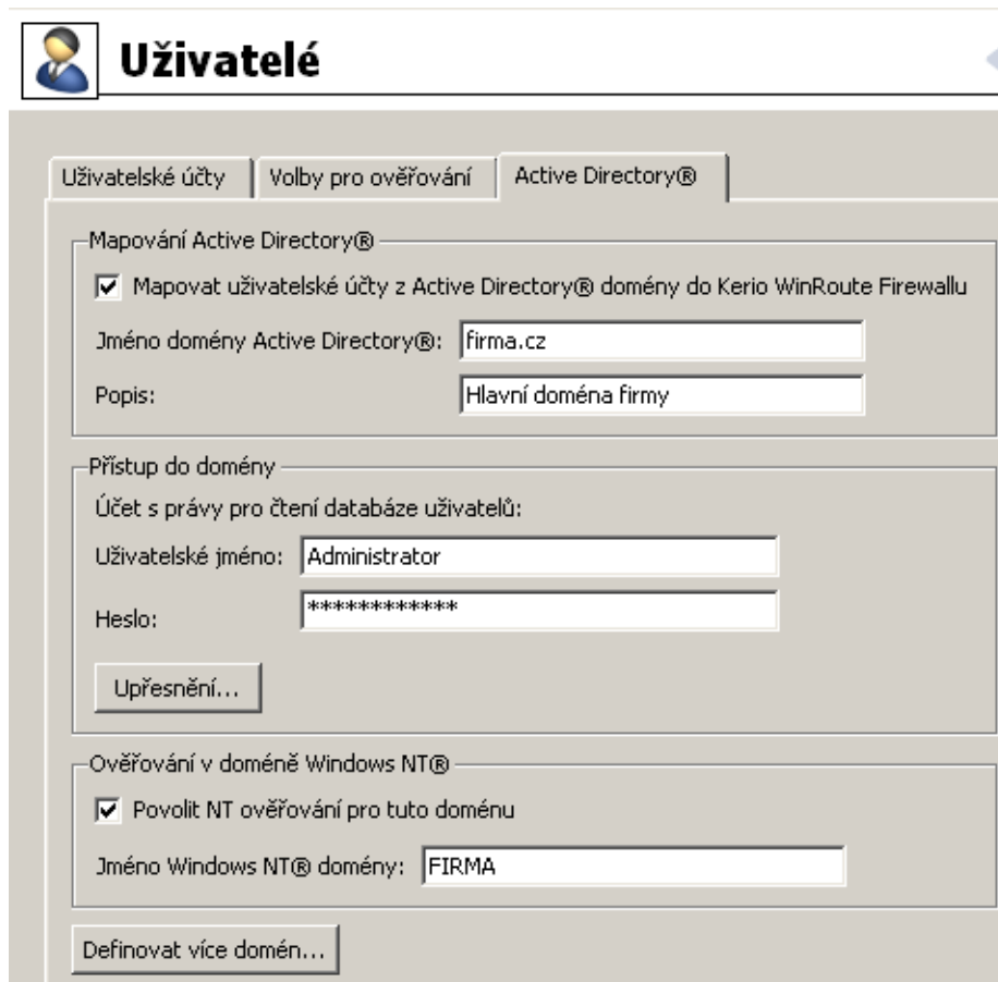
Obrázek 15.13 Mapování Active Directory domény
