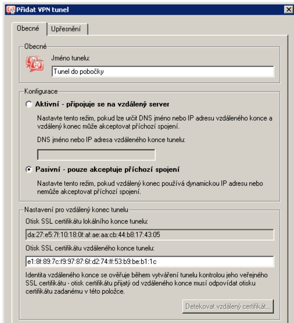
Obrázek 23.21 Centrála — definice VPN tunelu do pobočky
