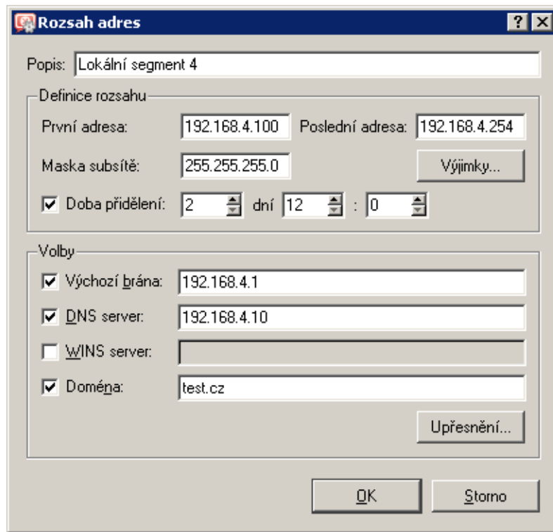
Obrázek 8.7 DHCP server — definice rozsahu adres
