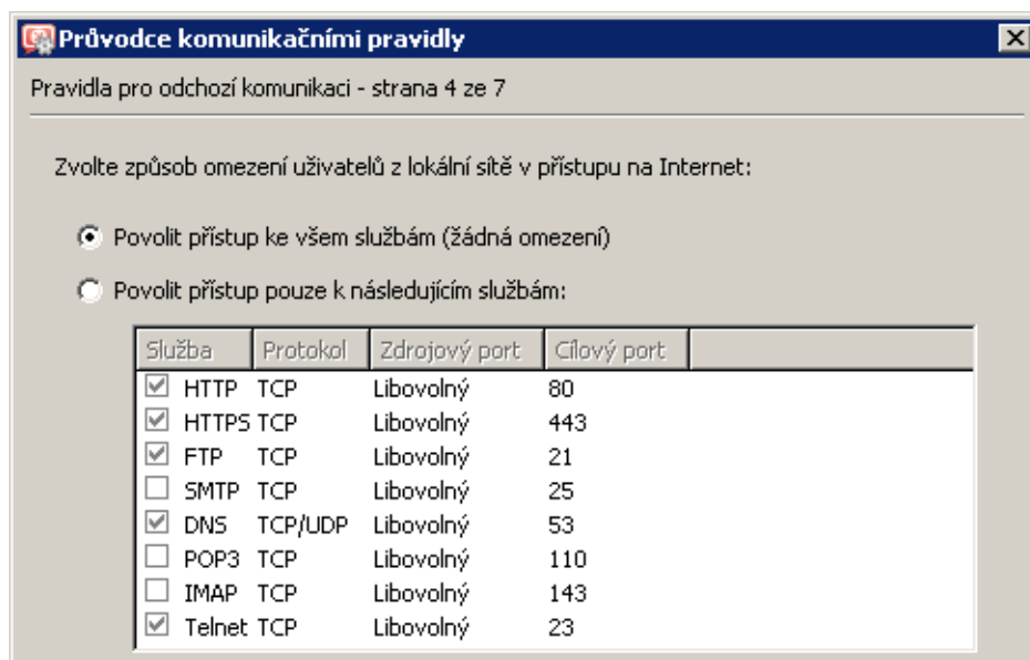
Obrázek 23.33 Centrála — přístup z lokální sítě do Internetu bez omezení
