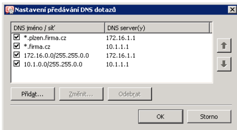
Obrázek 23.59 Pobočka Brno — nastavení předávání DNS dotazů
