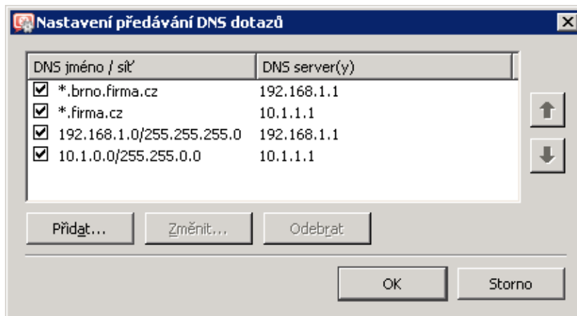
Obrázek 23.49 Pobočka Plzeň — nastavení předávání DNS dotazů
