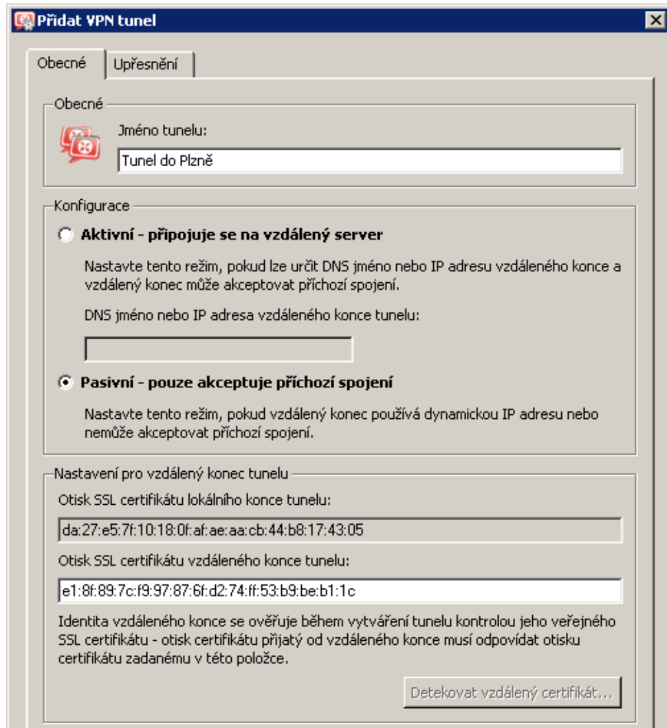
Obrázek 23.40 Centrála — definice VPN tunelu do pobočky Plzeň
